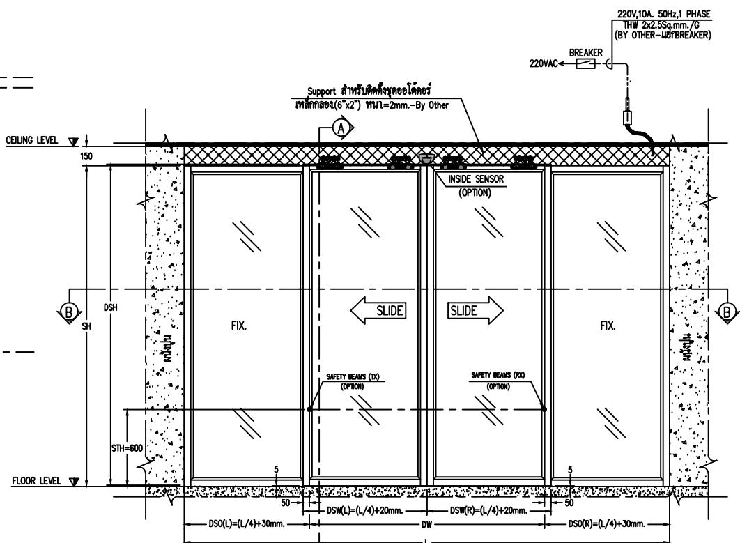
ELEVATION "C"
