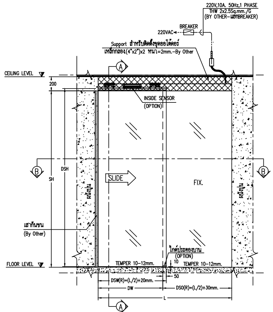
ELEVATION "C"
