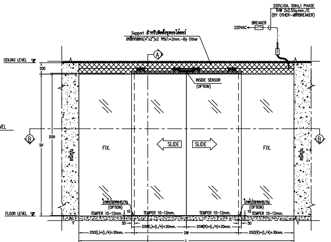
ELEVATION "C"
